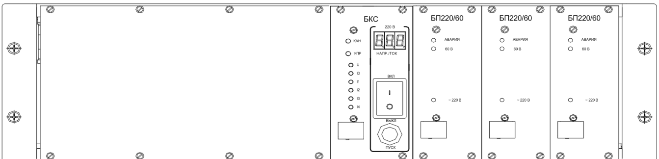
Рисунок 6 – Расположение ТЭЗ в МП-01
