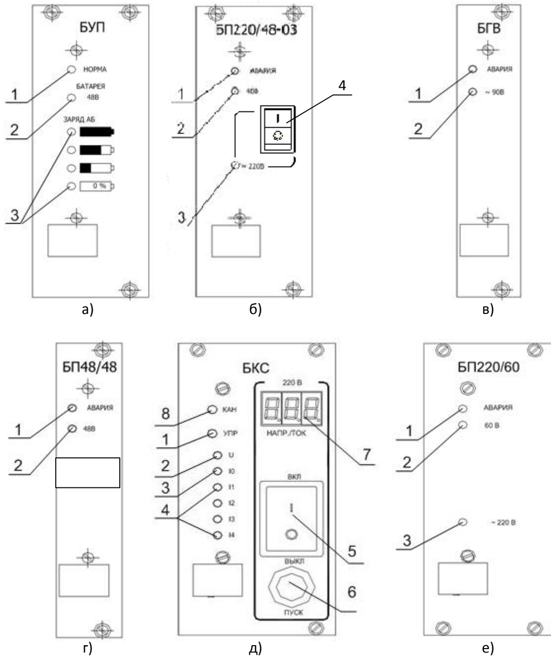
Рисунок 8 – Размещение органов управления, индикации и коммутации на передних панелях ТЭЗ исполнения 3U
