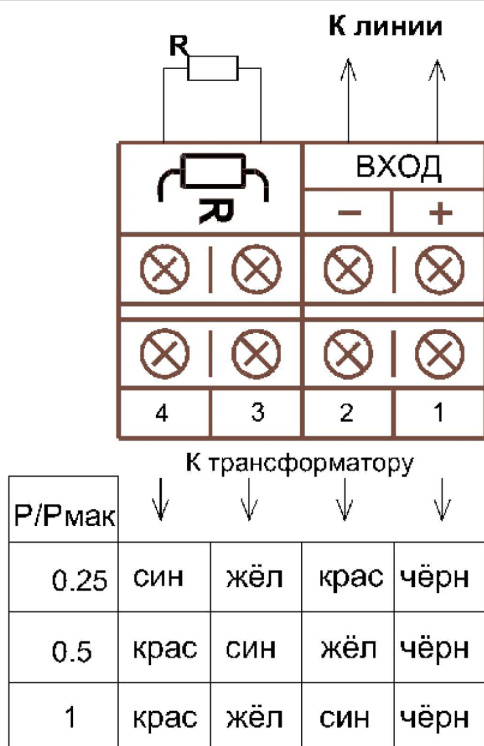
Рис.1. Схема подключения ОПР
